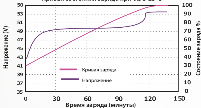
Кривая состояния заряда при 0.5C 25°C
