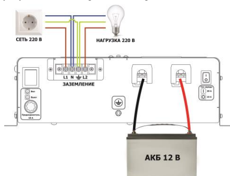
Рисунок 2 – Схема подключения ИБПС.
