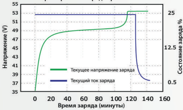
Графики состояния заряда при 25°C
