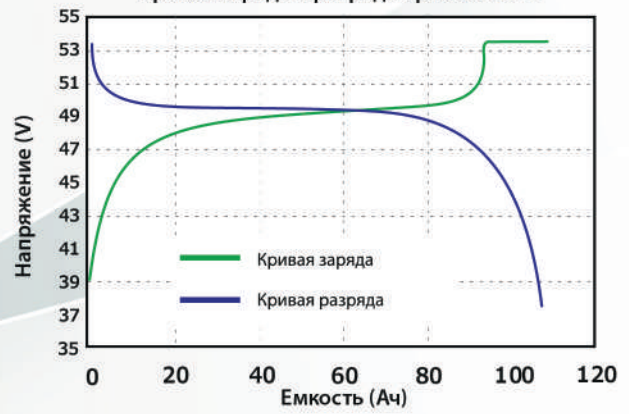
Кривая заряда и разряда при 0.5C 25°C
