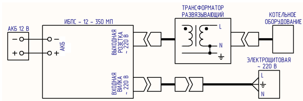
Рисунок 1 – Схема подключения ИБПС – 12 – 350 МП
